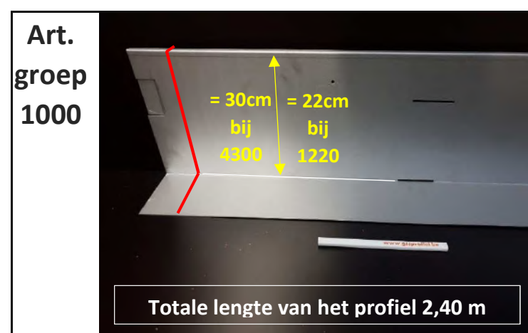
GSS-Profiel
