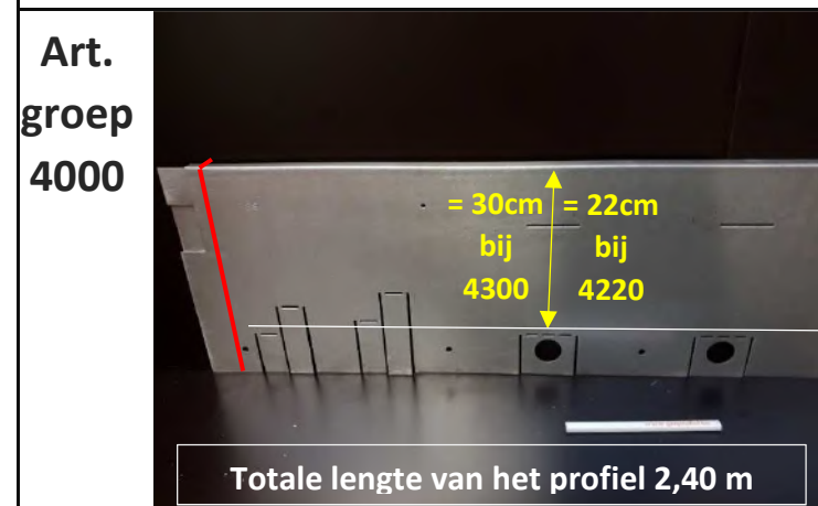
GSS-Balk
